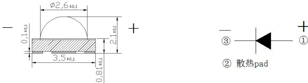
侧面图 120°
