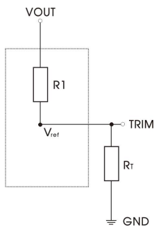
图 4 TRIM 的使用电路 (虚线框为产品内部)
