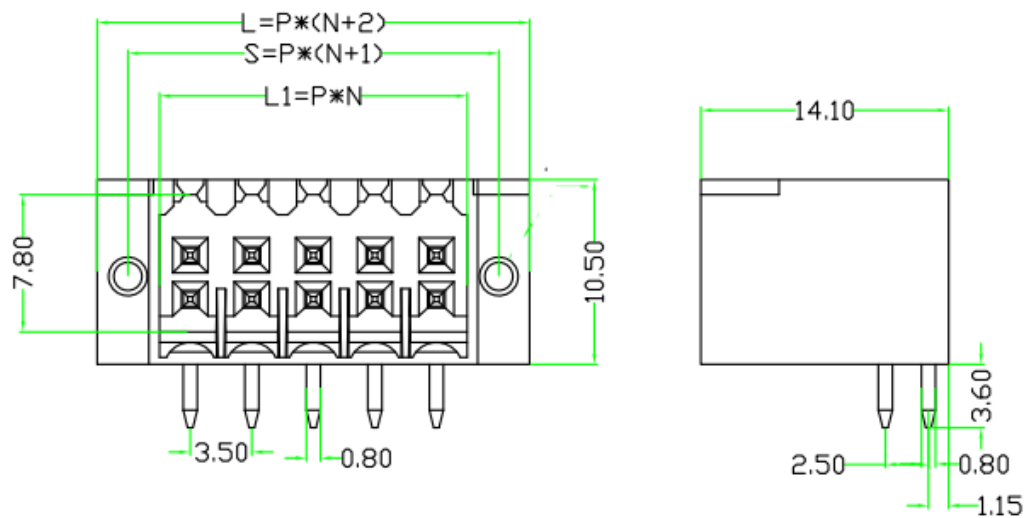
外形尺寸（Shape Dimension）
