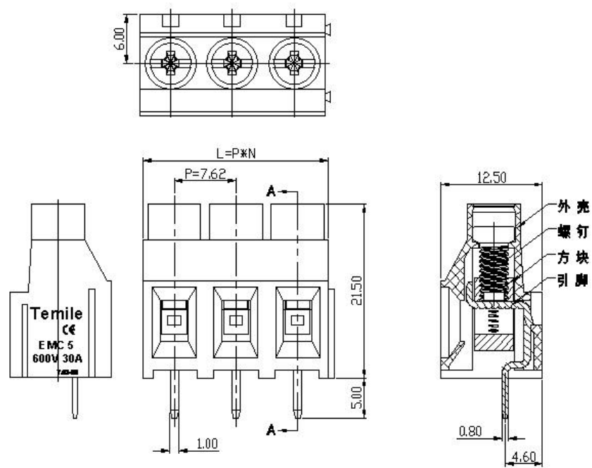
外形尺寸（Shape Dimension）
