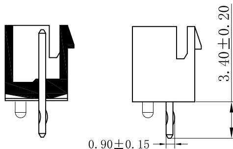
剖视图: A-A
