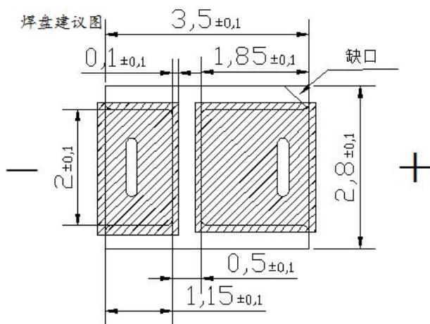
焊盘建议大小
