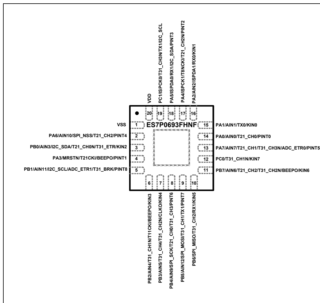
图 1-3 ES7P0693FHNF 顶视图
