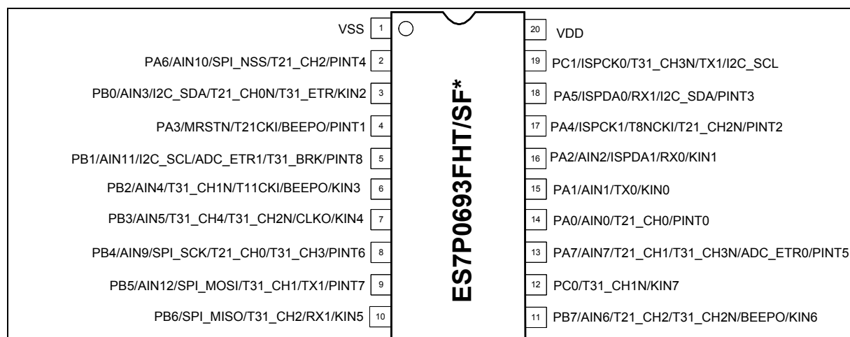
图 1-2 ES7P0693FHT/SF 顶视图
