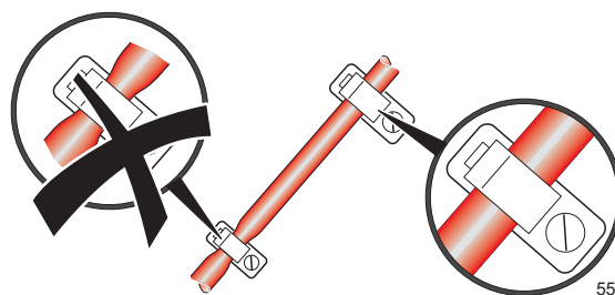
Figura 13 Utilizzare serracavi con ampie superfici di contatto (serracavi larghi)
