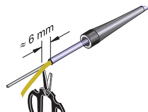
Figura 38 Tagliare lo scarico della trazione
