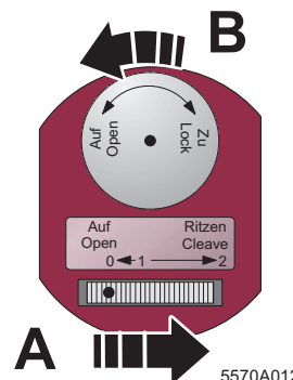
Figura 46 Rotella per l'incisione della fibra (A) e rotella per il serraggio della fibra (B)
