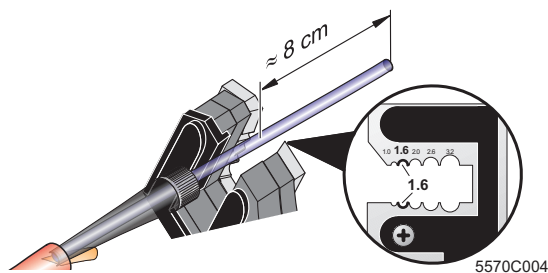
Figura 36 Spelare i conduttori singoli
