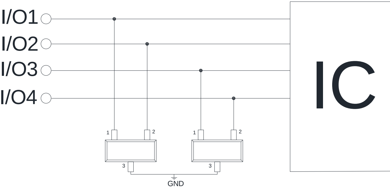
PESD2CANFD24LU-Q-ES
