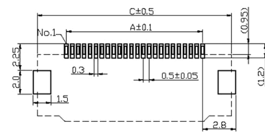
适用线路板 RECOMMENDED PCB LAYOUT
