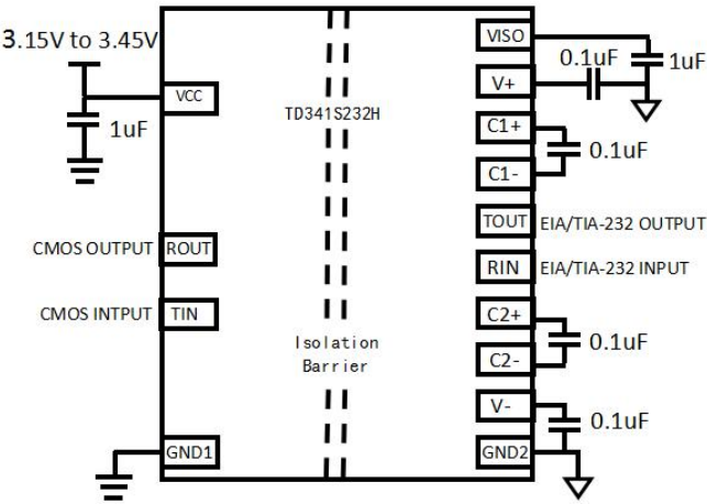
图 7. 典型应用电路
