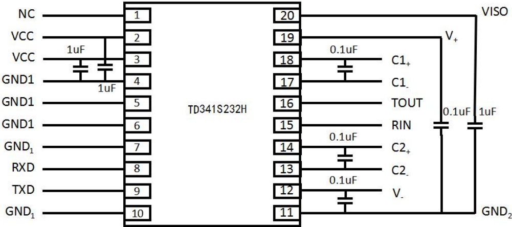
图 7. 典型应用电路
