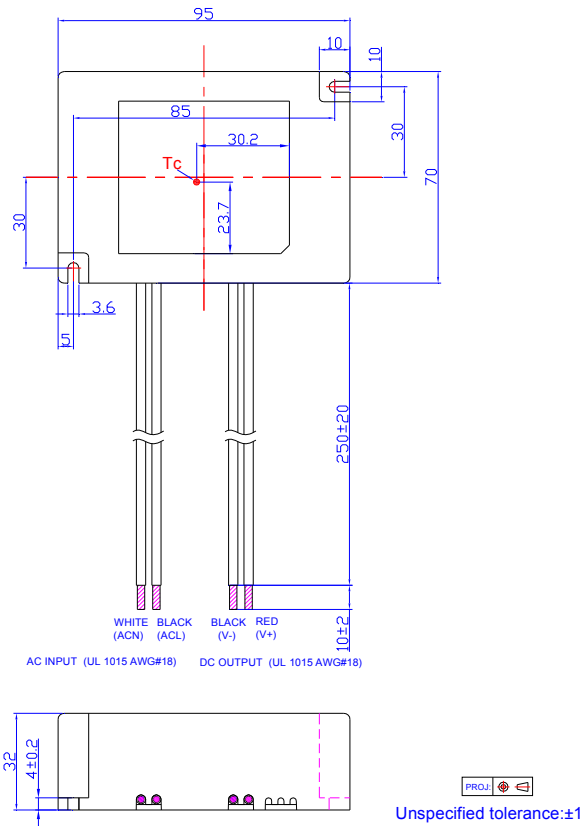
EUC-042SxxxPS
