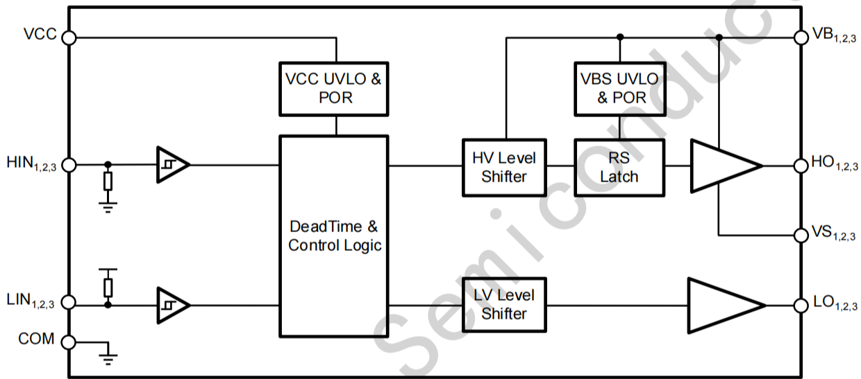
图 7-1 EG2134功能框图
