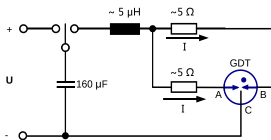
三极GDT回路（用于寿命试验）
