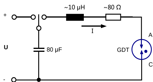
二极GDT回路（用于寿命试验）
