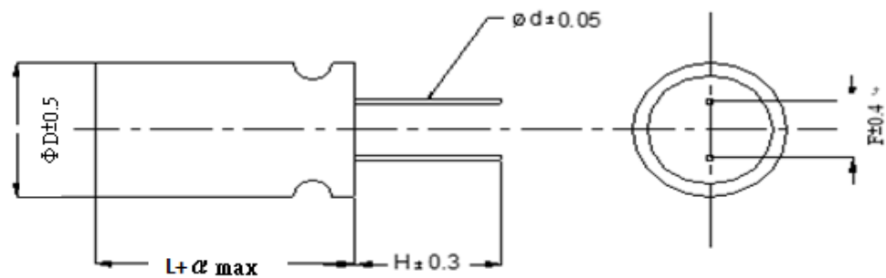
Fig. 2 Dimension
