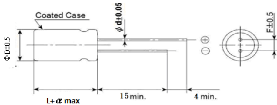
Fig. 2 Dimension
