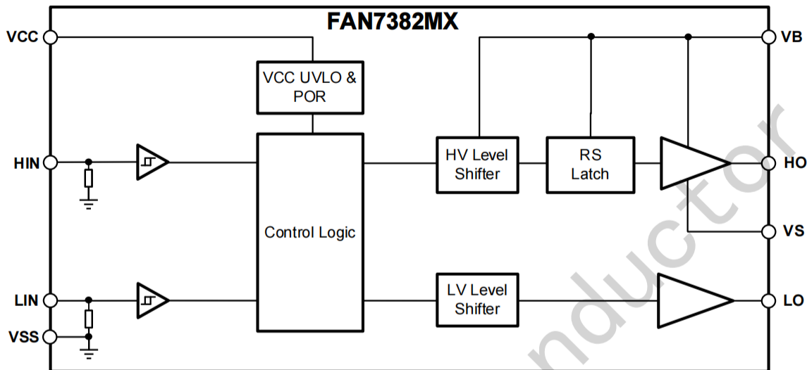
图 7 -1 FAN7382MX 的功能框图
