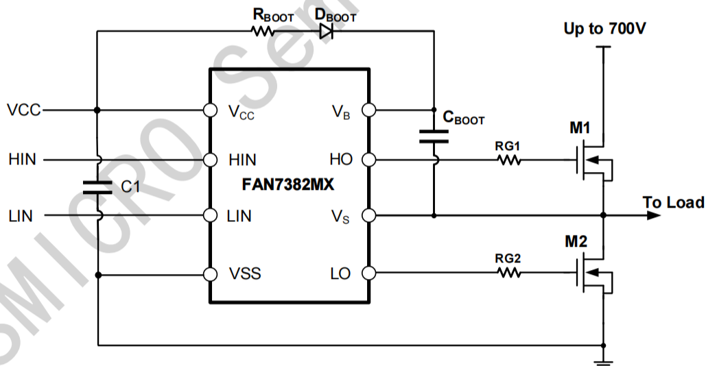
图 7 -2 FAN7382MX典型应用电路图
