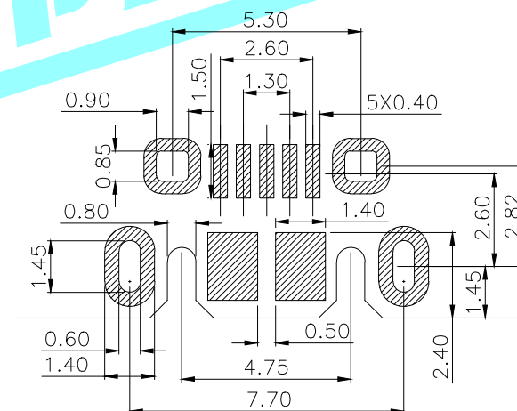
PCB LAYOUT PCB图仅做参考
