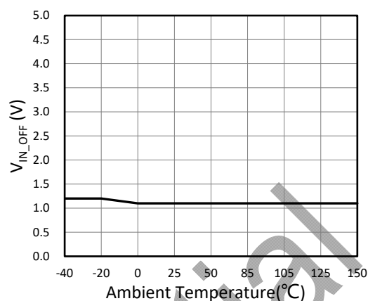
图 13 V_{IN\_OFF} VS. T_A
