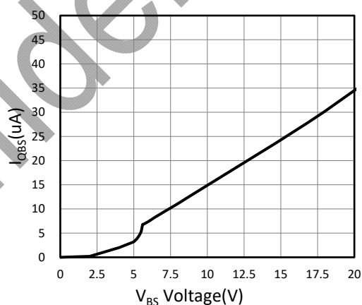
图 9 I_{QBS} vs. V_{BS}
