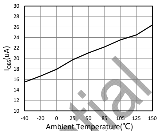
图 7 I_{QBS} vs. T_A
