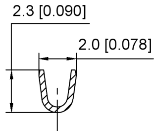
SEC:A-A
