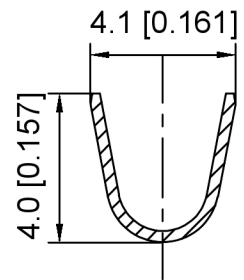
SEC:B-B
