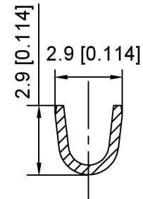
SEC:A-A
