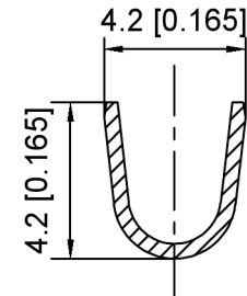
SEC:B-B
