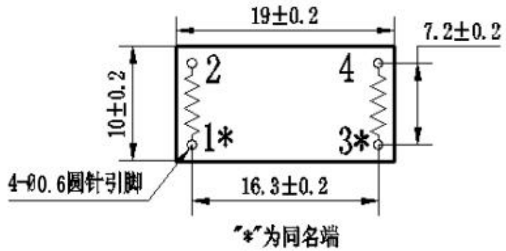
底视图
