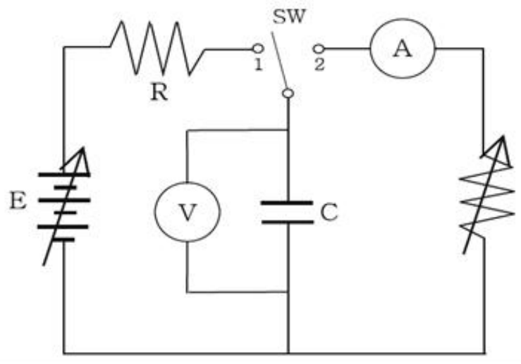
图1 容量测试电路图
