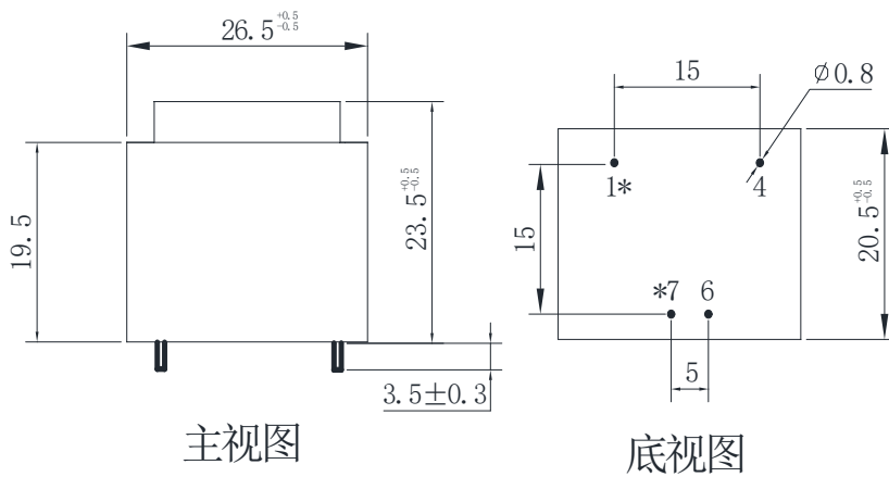
外形尺寸图 (mm)
