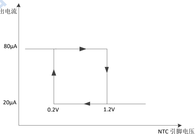
图 19 NTC 电压和放出电流关系
