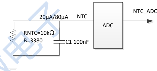
图 18 电池 NTC 比较
