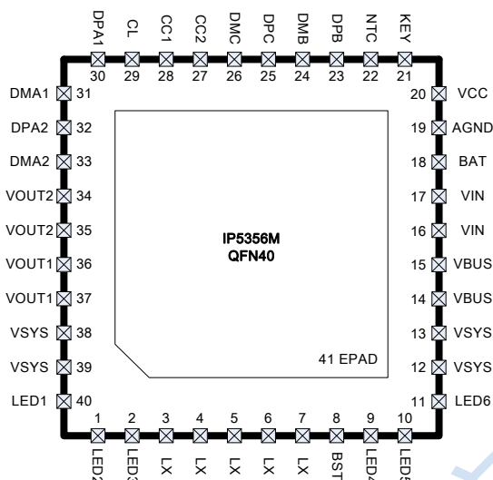
图 2 IP5356M 引脚图
