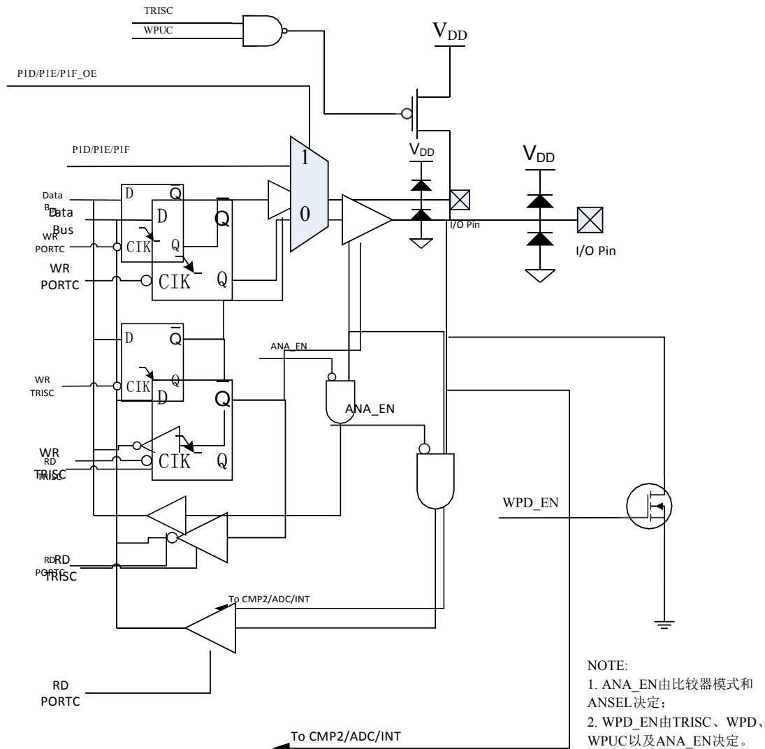
图 16.8 PC0, 1, 2 架构框图
