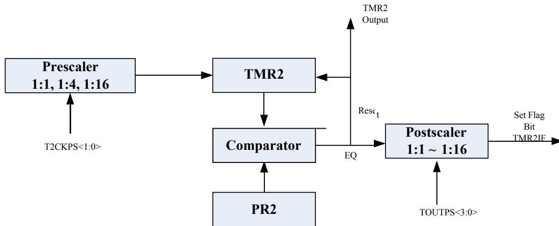
图 8.1 定时器 2 框图
