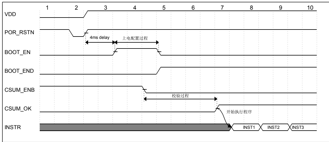
图 4.4 校验过程
