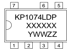
DIP-7
