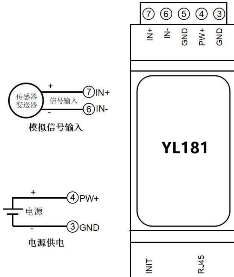
图 3 YL181 模块接线图
