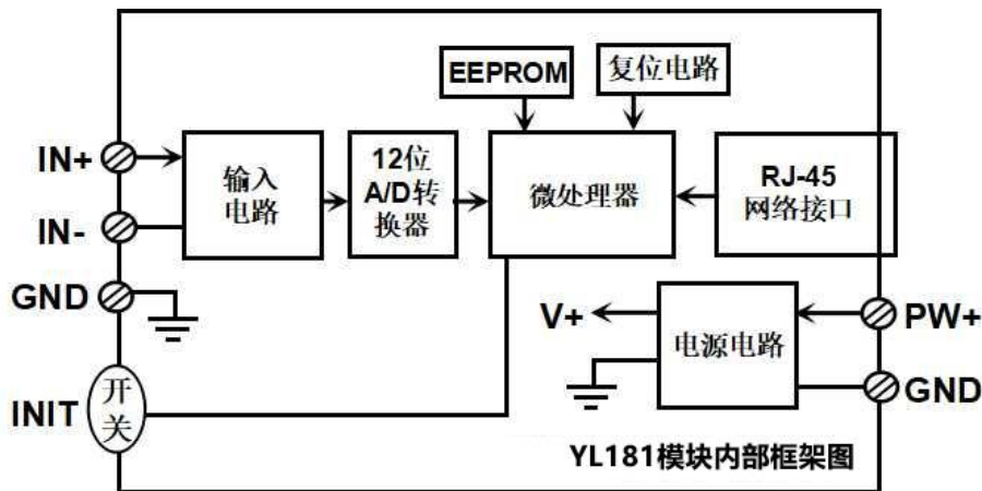
图2 YL181 模块内部框图
