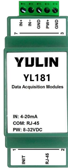
图1 YL181 模块外观图
