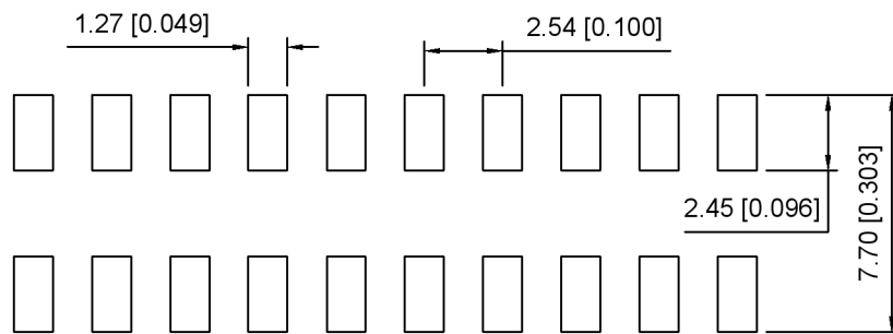
P.C.B LAYOUT
