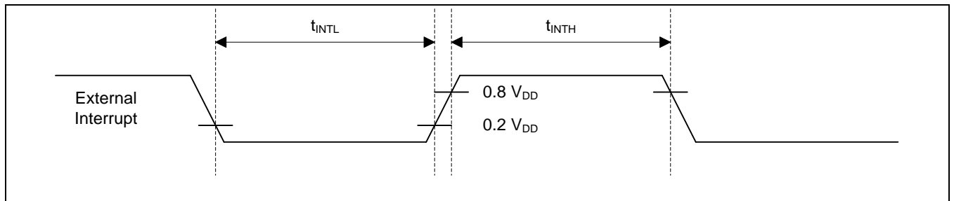
Figure 24-3 外部中断输入时序
