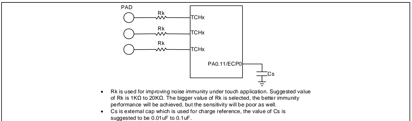
Figure 23-2 Touch Sensor应用连接图
