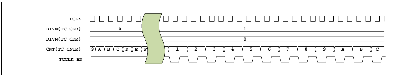
Figure 14-3 2分频的计数器时序图
