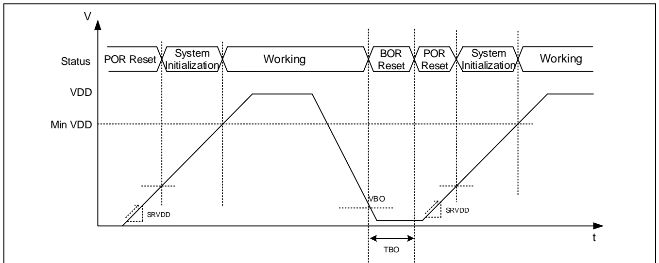
Figure 24-2 上电和掉电示意图
