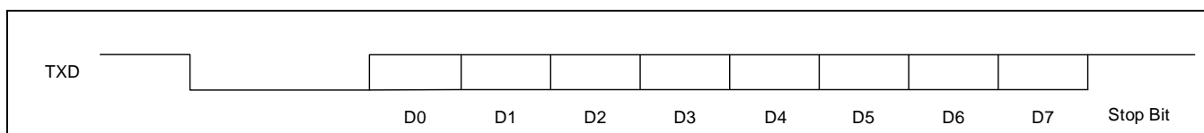
Figure 13-4 数据发送
