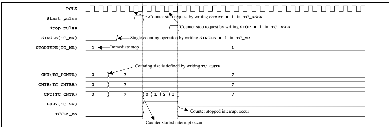
Figure 14-15 立即停止的时序图，例2 (单次计数，有停止请求)
