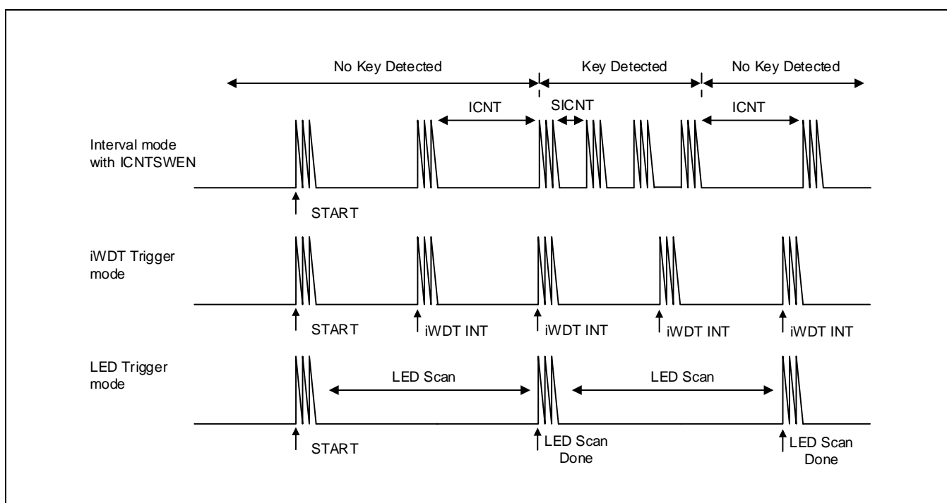
Figure 23-5 自动扫描模式
