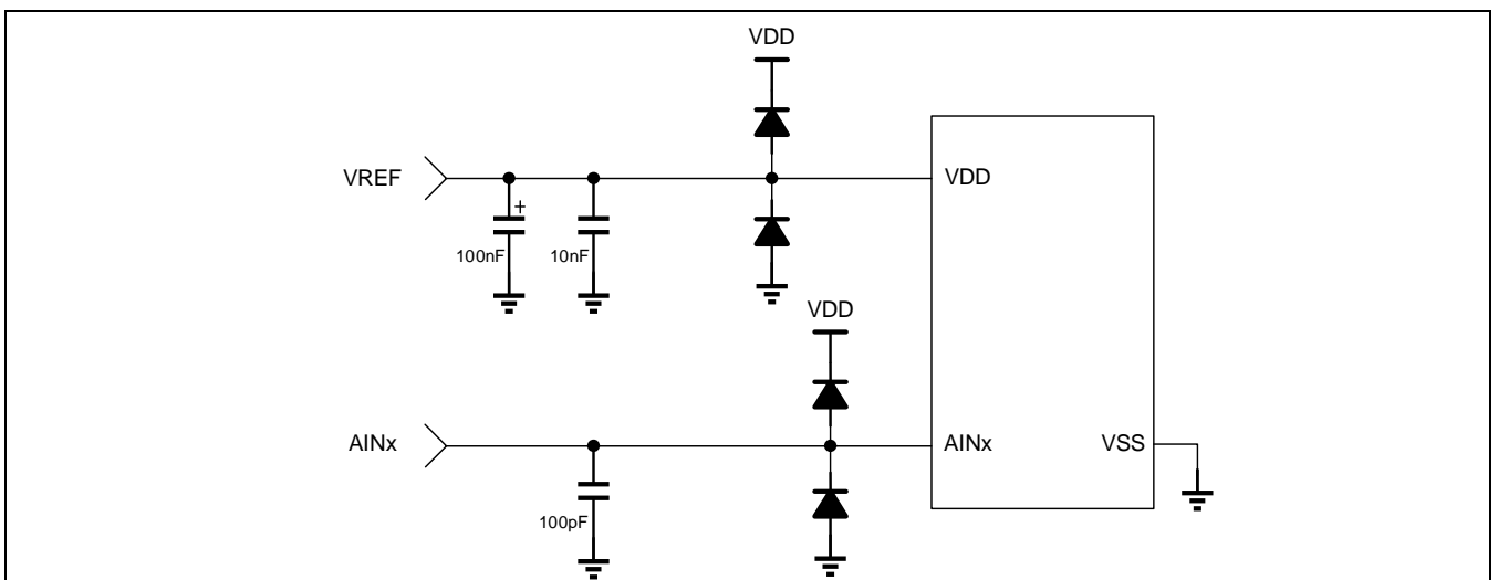
Figure 8-2 参考电路
