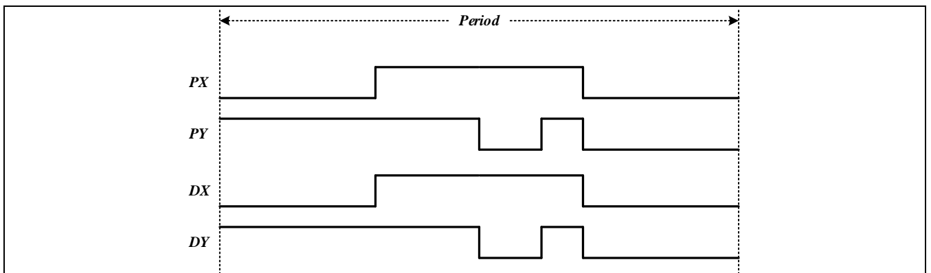
Figure 16-21 死区控制示例1: BYPASS 模式，PX和PY直接输出
