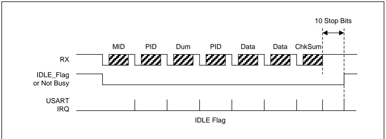
Figure 18-6 空闲标志
