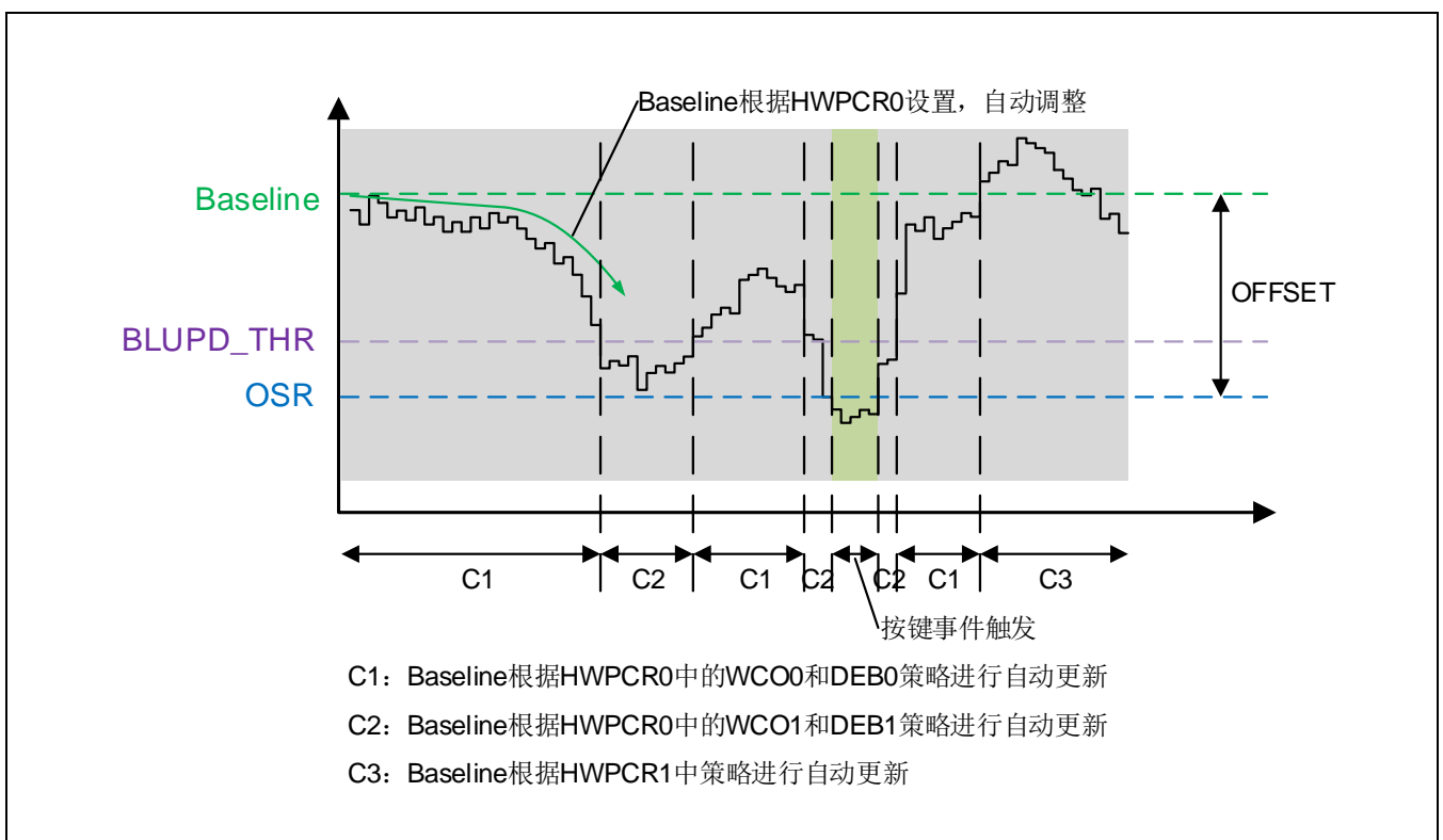
Figure 23-4 按键触发示意图
