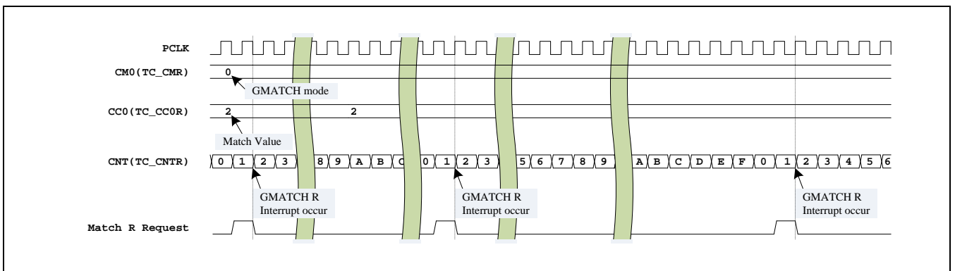
Figure 14-18 通道0的匹配模式时序图例
