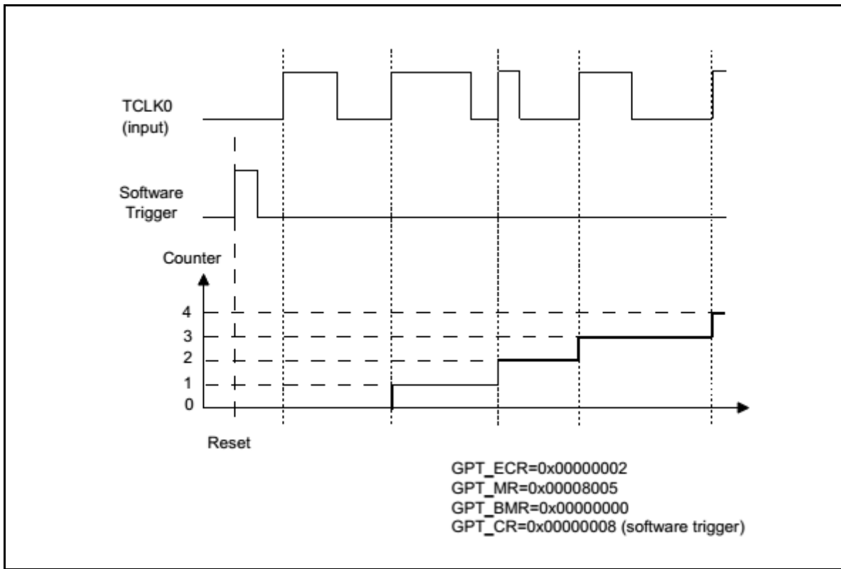
Figure 12-13 事件计数
