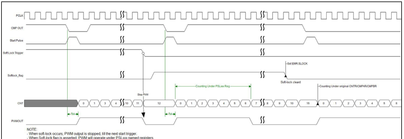
Figure 16-11 Soft Lock 普通模式
