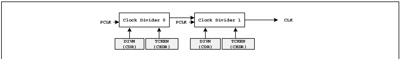
Figure 14-2 时钟控制模块框图
