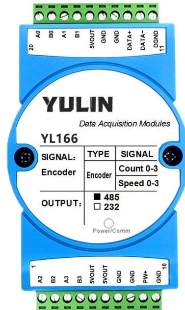
图1 YL166 模块外观图
