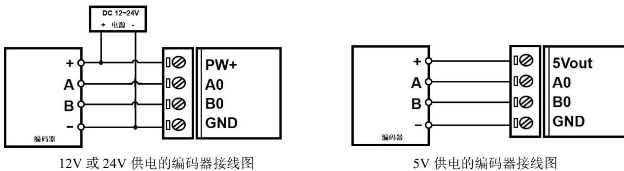
图3 YL166 模块接线图
