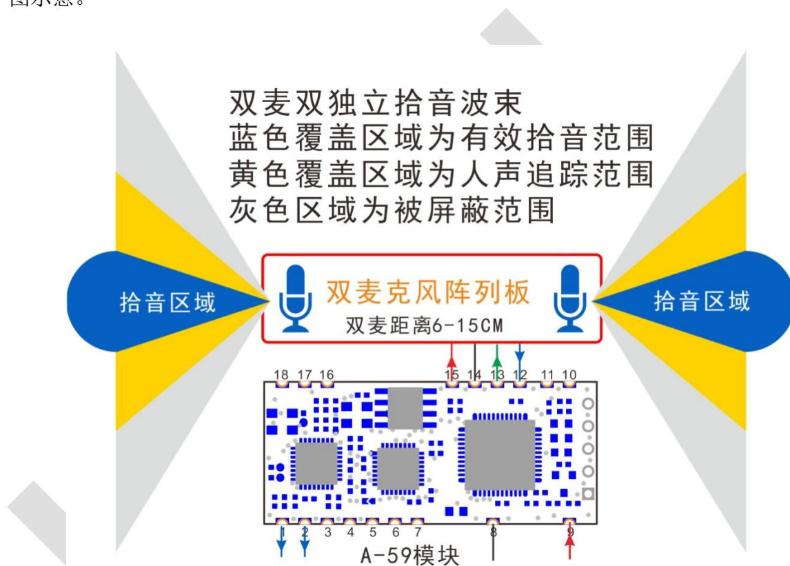
A-59 模块配合双麦克风的双拾音波束示意图
