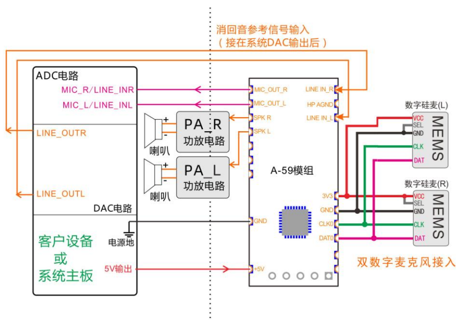
功放接在模组之后连接图（消回音模式二）
