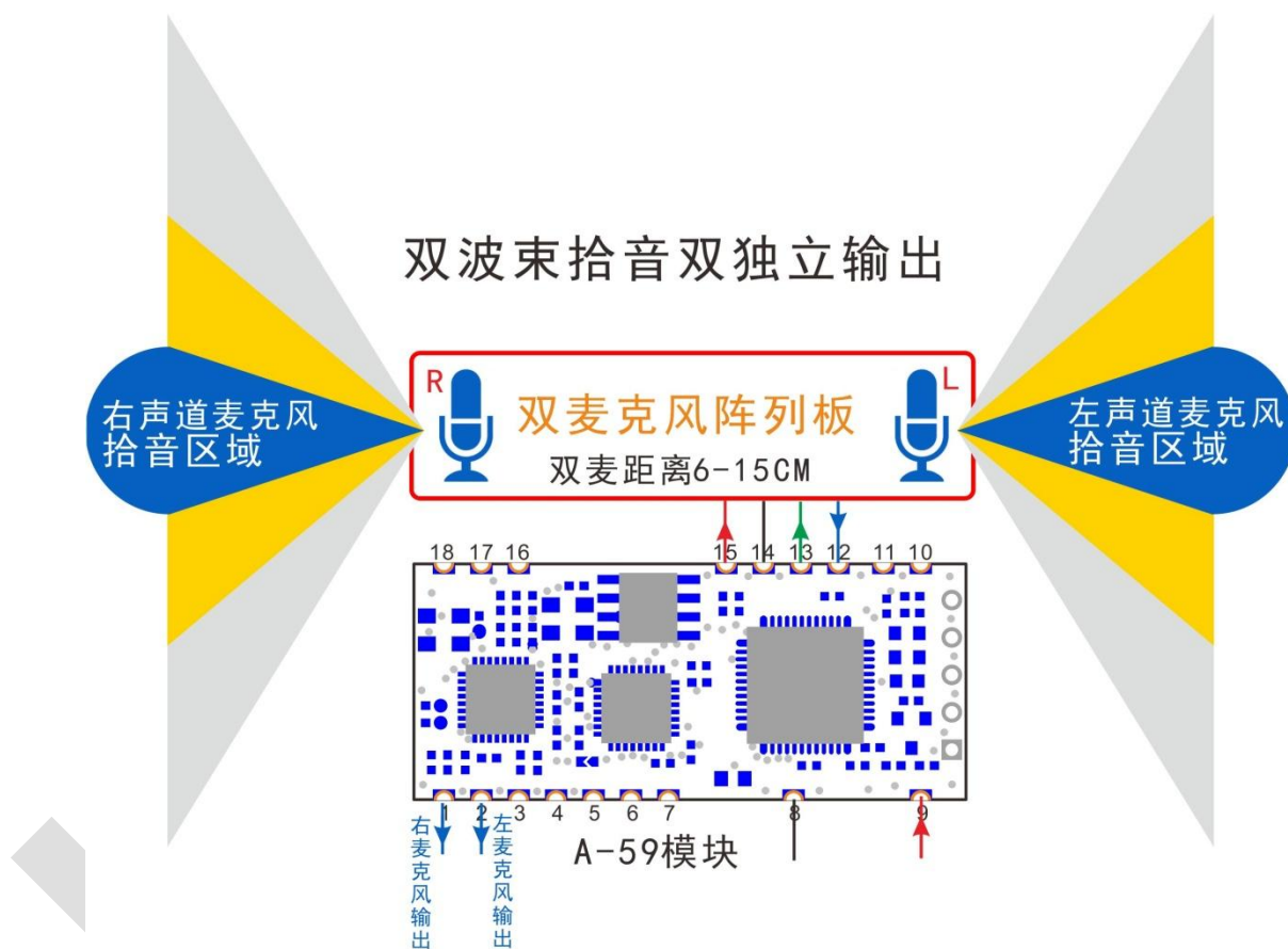
A-59 模块双麦克风双通道音频输出示意图
