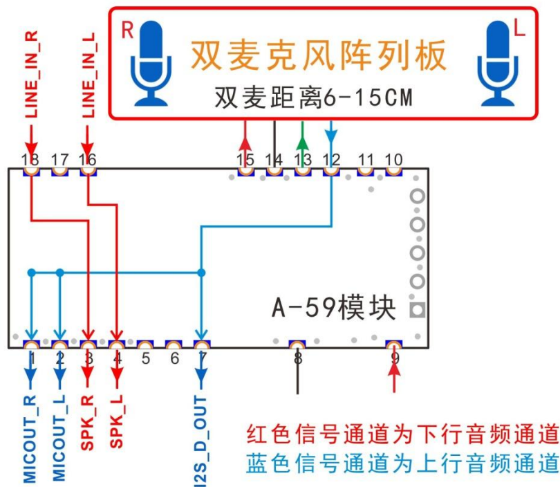
A-59 模组内部音频通道图示
