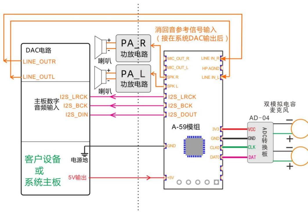
数字音频输出功放接在模组之后连接图（消回音模式八）
