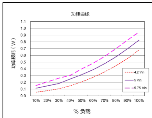
功耗曲线 ( V_{out}=3.7V )
