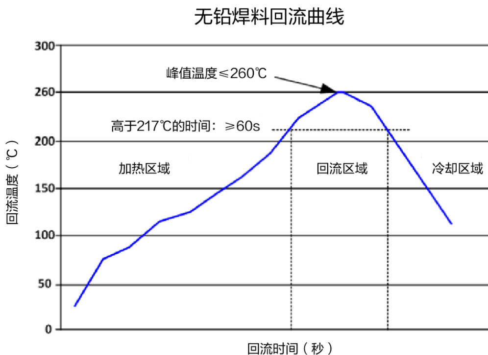
图 9-1 推荐无铅焊料回流曲线
