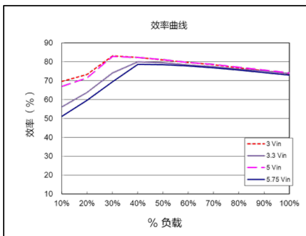
效率曲线 ( V_{out}=0.8\text{V} )
