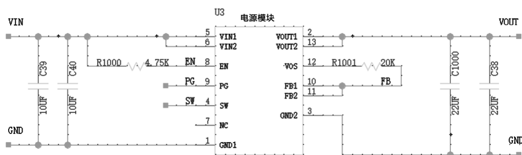
图 4-1 推荐应用电路
