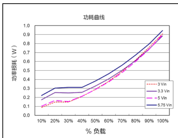
功耗曲线 (V out =1.2V)
