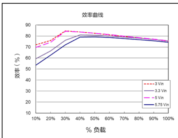
效率曲线 ( V_{out}=0.9\text{V} )
