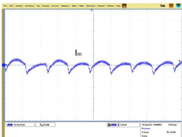
输入反射纹波电流
