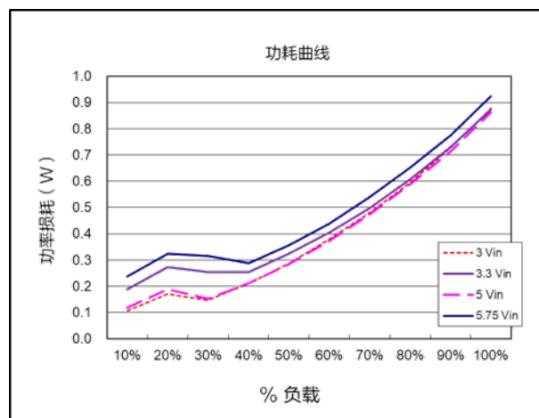
功耗曲线 ( V_{out}=0.9\text{V} )
