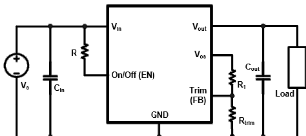
图 4-3 应用电路图
