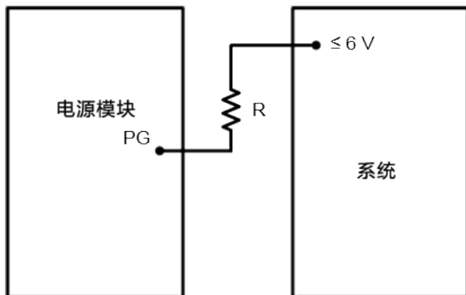
图 5-6 保护组配置图
