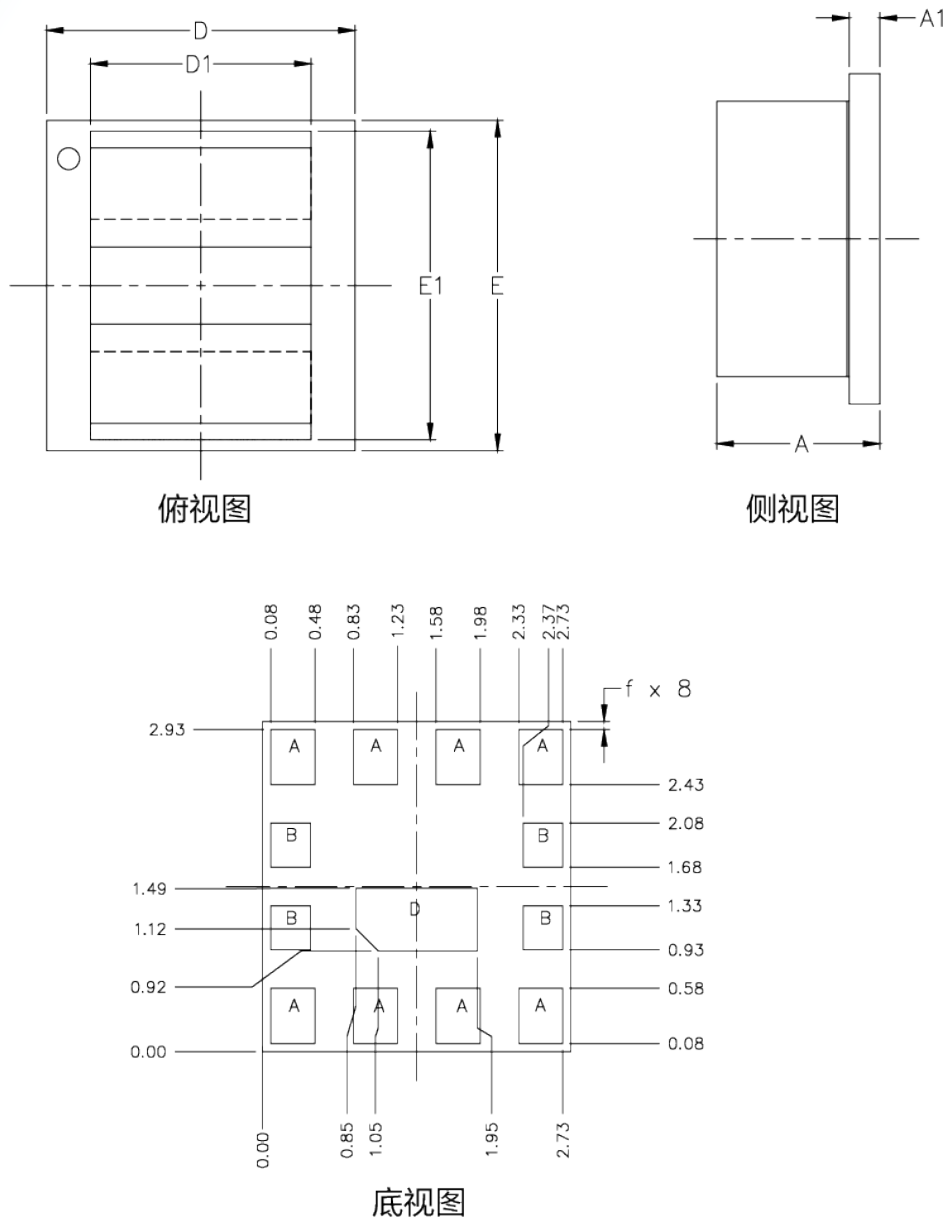
图 5-2 结构尺寸图
