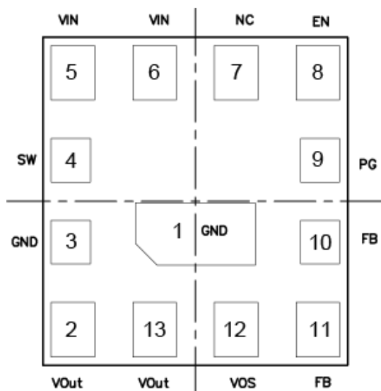
图 5-3 引脚说明
