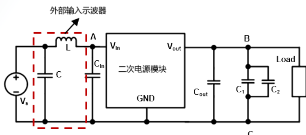
图 4-2 测试电路图
