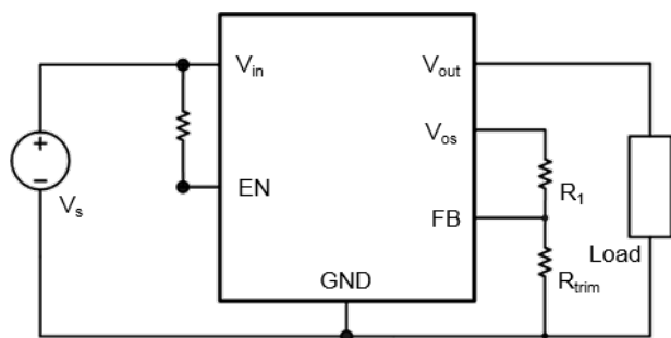
图 5-5 R trim 外部连接
