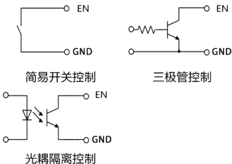
图 5-4 EN 引脚控制方式推荐图
