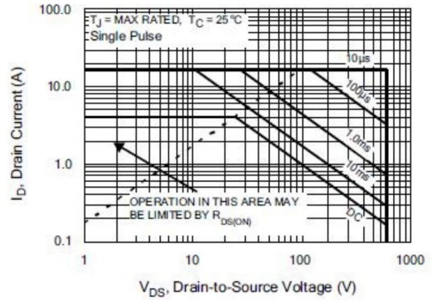
图 6-2 SIF5N65F(TO-220FP(L))
