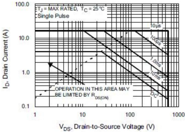
图 6-1 SIF5N65F(TO-220)
