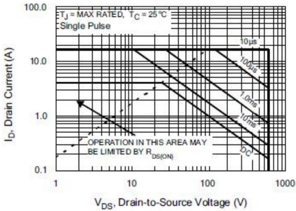
图 6-3 SIF5N65F(TO-262&263)
