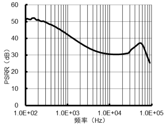
图 2.8 PSRR 与频率关系 ( I_{OUT}=1mA )
