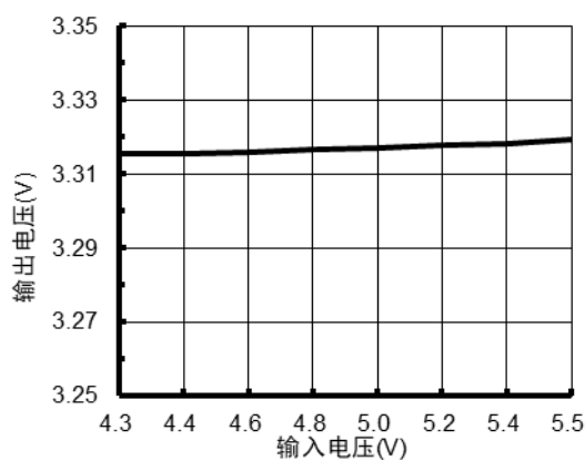
图 2.6 线性调整特性
