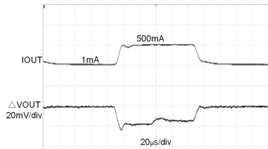
图 2.10 负载瞬态响应波形
