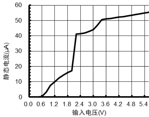
图 2.4 输入电压与静态电流关系
