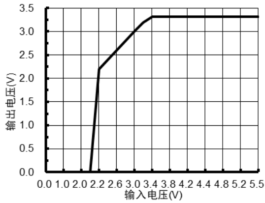
图 2.2 输入电压与输出电压关系
