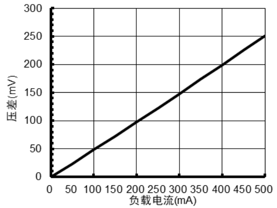
图 2.3 压差与负载关系
