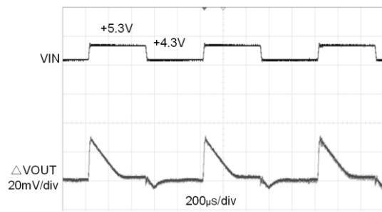
图 2.9 线性瞬态响应波形
