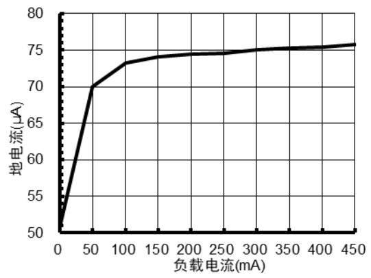
图 2.5 负载电流与地电流关系
