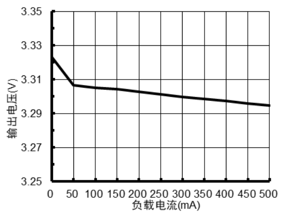
图 2.7 负载调整特性
