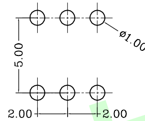
印刷电路板焊接处尺寸图
