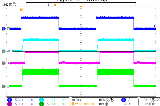
Figure 13. EN toggle (Iload=6A)
