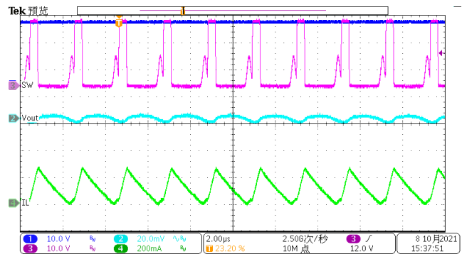
Figure 20. Output Ripple (Iload=100mA)
