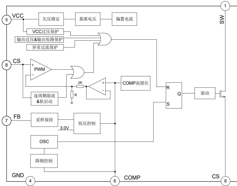
DC/DC部分
