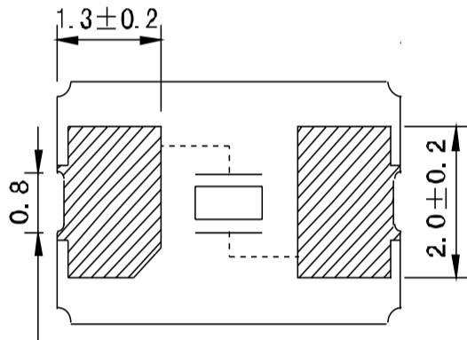
(Bottom View) 仰视图
