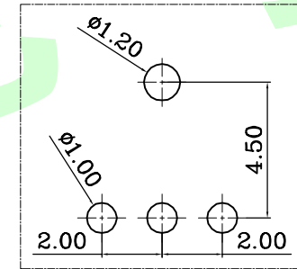
印刷电路板焊接处尺寸图
