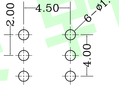
印刷电路板焊接处尺寸图
