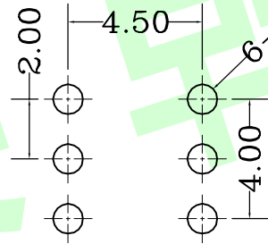
印刷电路板焊接处尺寸图
