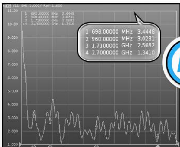
■ 某吸盘天线电压驻波比大于1.5
