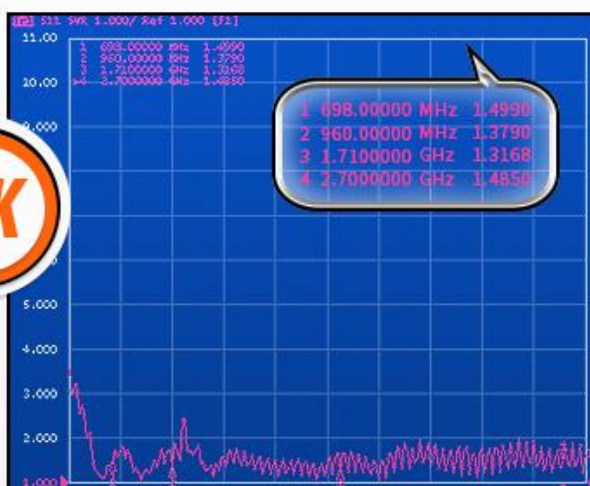
■ 我司吸盘天线电压驻波比值
