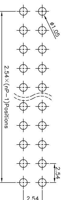
P.C.B LAYOUT
