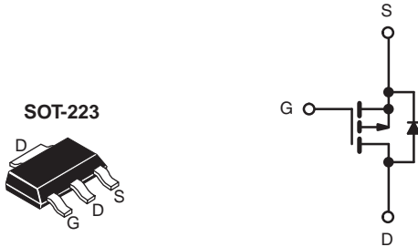
P-Channel MOSFET
