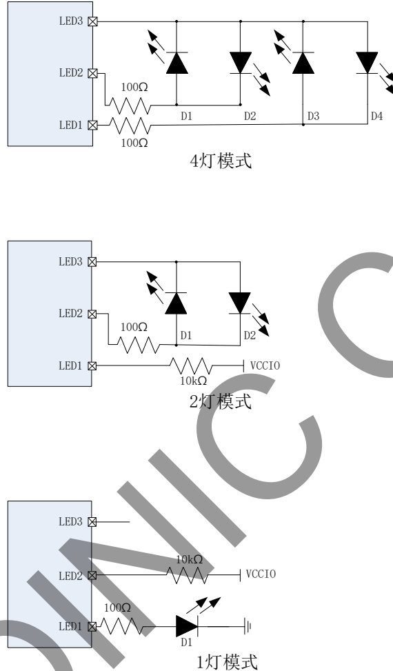
图 11 4 颗、2 颗、1 颗 LED 连接方式
