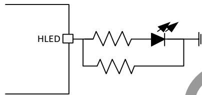
图 9 快充指示灯电路
