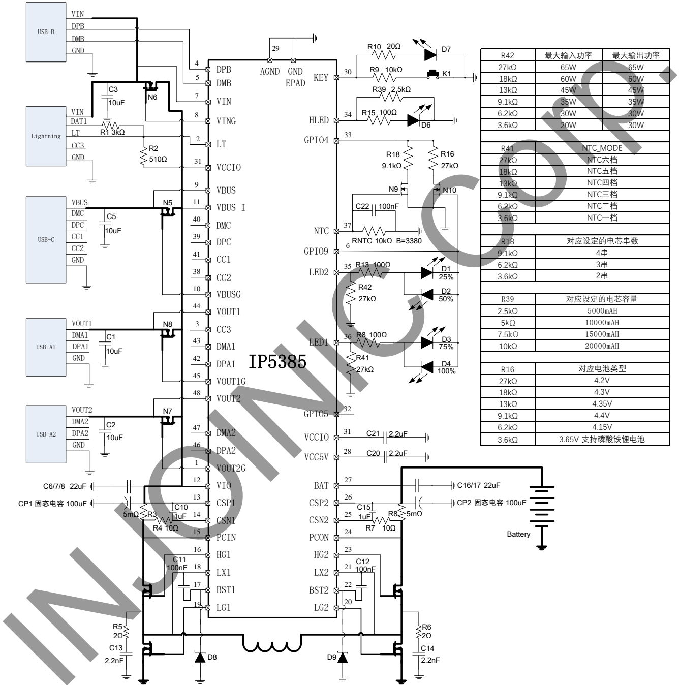
图 22 IP5385 LED 应用原理图
