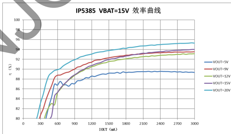
图 4 4 串 65W 放电效率曲线图
