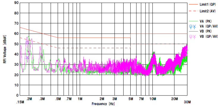
Figure 24. V_{IN} : 115 Vac / 60 Hz, I_{OUT} : 2 A
