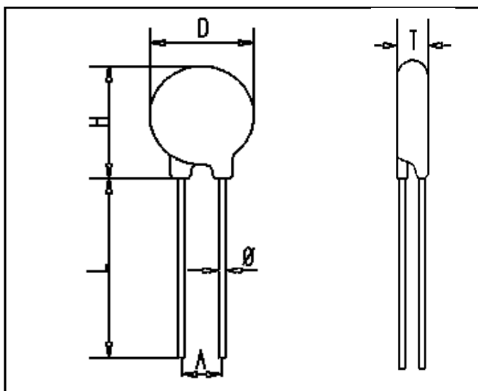
外观尺寸图 (单位 Unit:mm)
