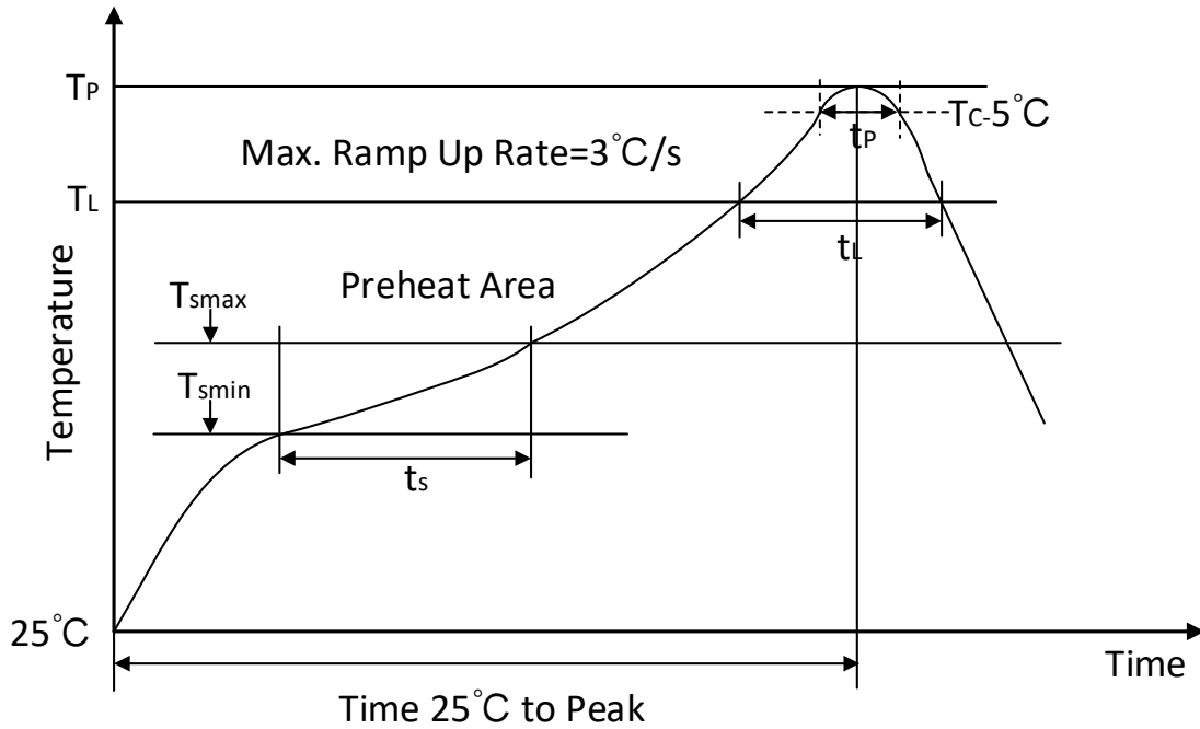
图 12-1 焊接温度曲线
